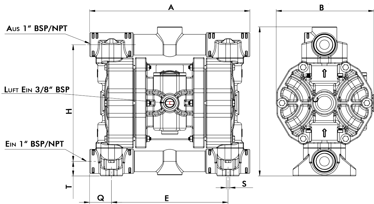
Abmessungen [mm]
