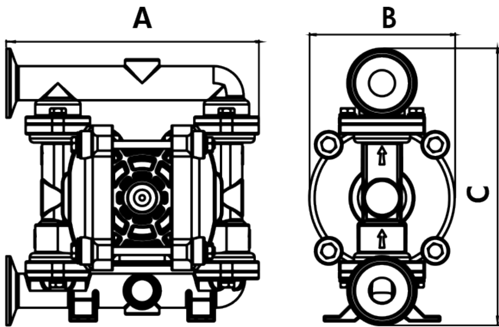
Abmessungen [mm]
