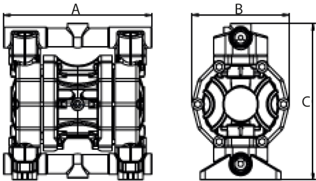
Abmessungen [mm]
